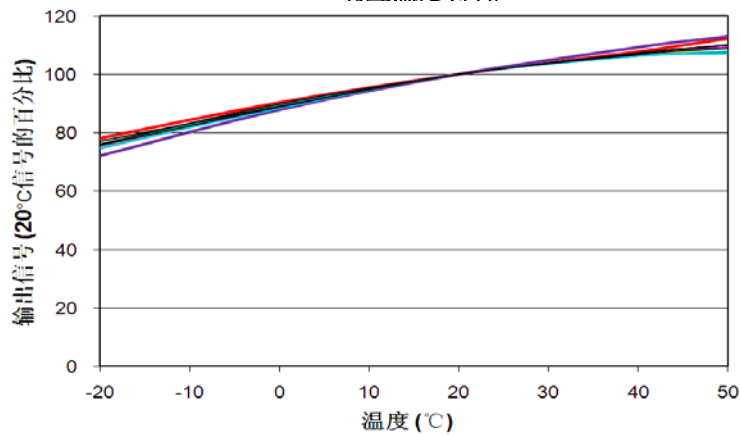
响应温度特性
