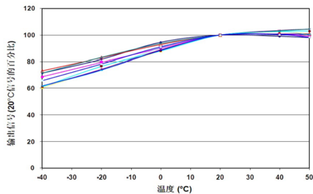
响应温度特性
